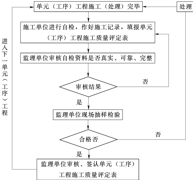
图 1 单元工程质量检验工作程序图
